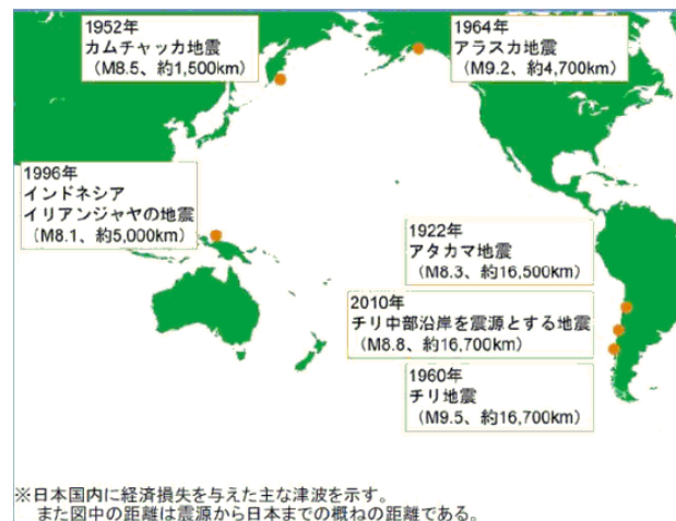
遠地津波の要因となる主な地震
